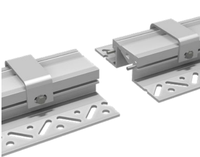
FS 75/42 (einteilige Profilkonstruktion)
