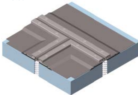
T-Stück IF
