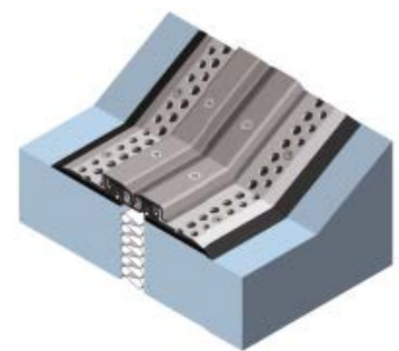
Gefälleendpunkt
