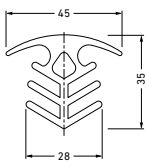
FA 15/4535 Material: PVC Fugenbreite max.: 20 mm
