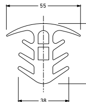
FA 15/5538 Material: PVC Fugenbreite max.: 25 mm
