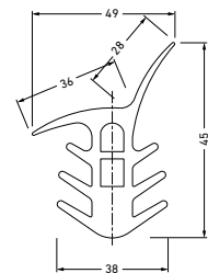
FAE 15/3638 (für Eckfugen) Material: PVC Fugenbreite max.: 25 mm
