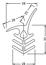
FAE 15/3035 (für Eckfugen) Material: PVC Fugenbreite max.: 20 mm
